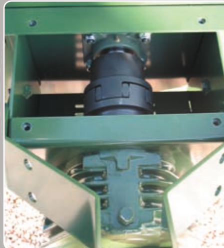
Trasmissione per versione a trattore Transmission for tractor version Transmission pour version à tracteur Antrieb für Traktor Version Transmisión y para versión para tractor Transmissie voor tractor aangedreven versie
